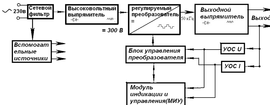
Рисунок 1.2 – Структурная схема источника питания
